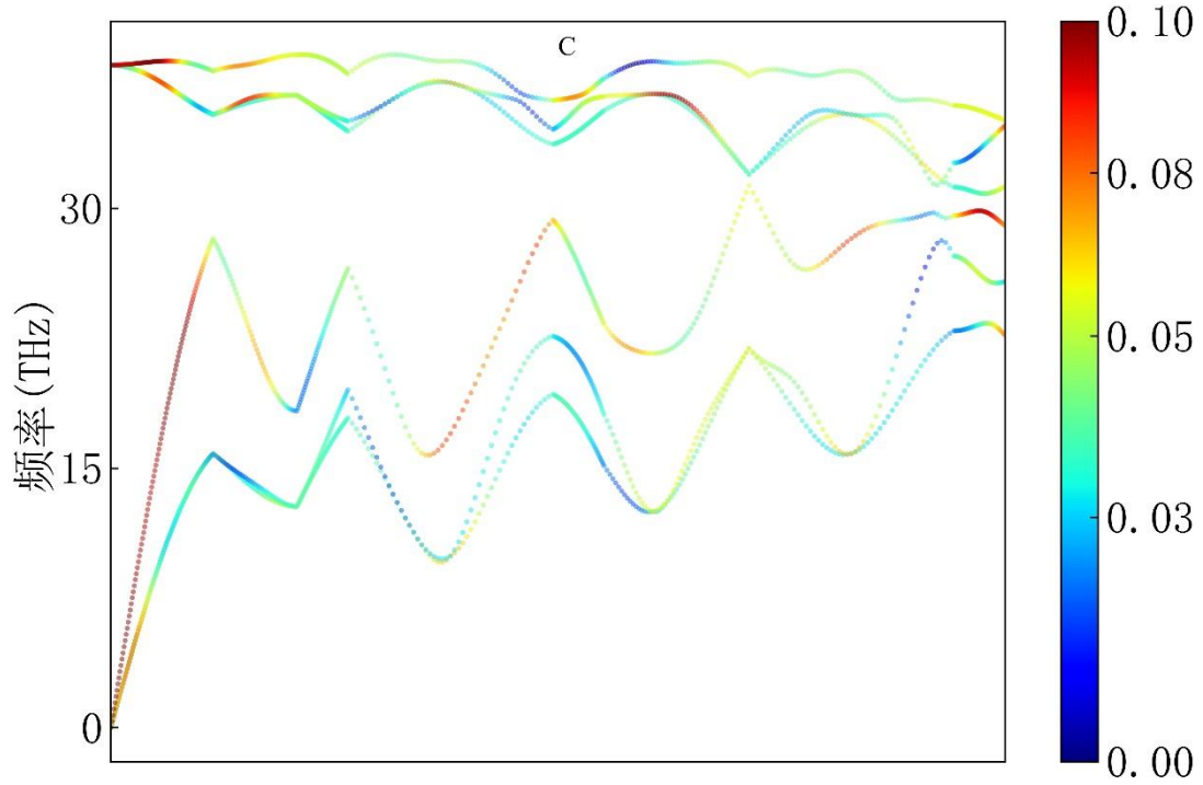
图 S2 C 晶体的声子谱，图中点的颜色值为对应声子模式的非简谐性描述符 \sigma_{q,j}^A
