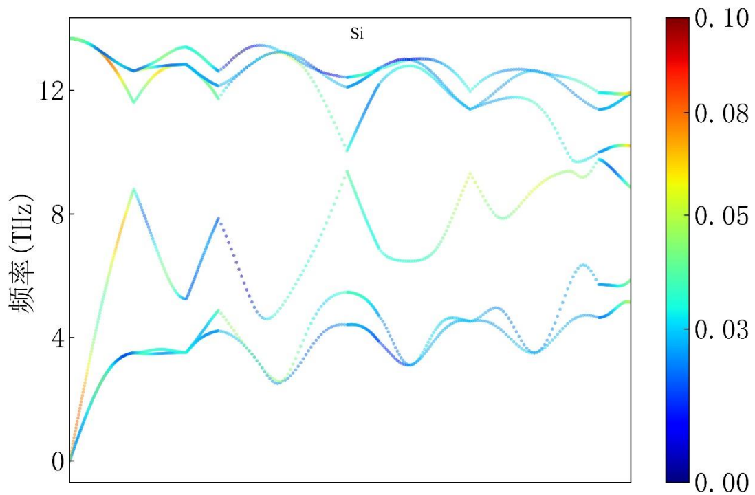
图 S3 Si 晶体的声子谱，图中点的颜色值为对应声子模式的非简谐性描述符 \sigma_{q,j}^A
