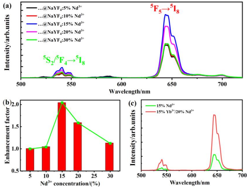
图 S3 在 800 nm 近红外光激发下, \text{NaYF}_4:20\% \text{Yb}^{3+}/12\% \text{Ce}^{3+}/2\% \text{Ho}^{3+}@\text{NaYF}_4:x\% \text{Nd}^{3+} ( x = 5, 10, 15, 20, 30 )核壳纳米晶体的(a)上转换发射光谱和(b)增强因子, (c) \text{NaYF}_4:20\% \text{Yb}^{3+}/12\% \text{Ce}^{3+}/2\% \text{Ho}^{3+}@\text{NaYF}_4:15\% \text{Nd}^{3+} 和 \text{NaYF}_4:20\% \text{Yb}^{3+}/12\% \text{Ce}^{3+}/2\% \text{Ho}^{3+}@\text{NaYF}_4:15\% \text{Yb}^{3+}/20\% \text{Nd}^{3+} 核壳纳米晶体的上转换发射光谱
